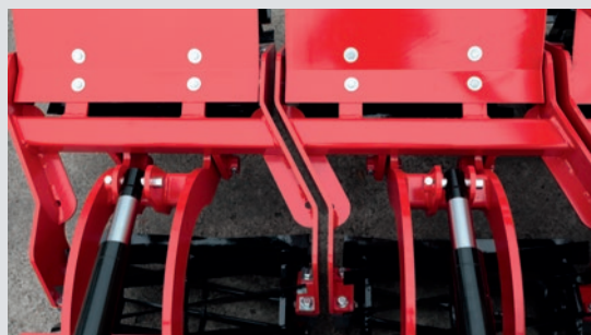
Z-förmig versetzte Reihen vermeiden Lücken zwischen den Walzenabschnitten
